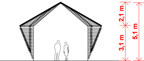
CARBET TYPE - COUPE AA'
