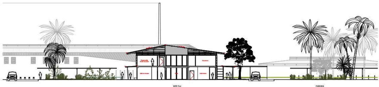
COUPE AA' SPIP-PJJ
