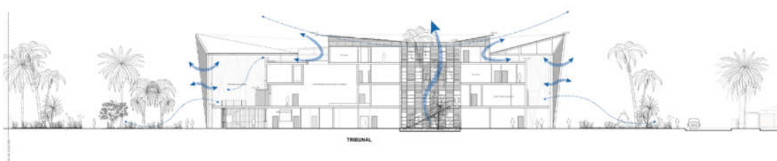
Ventilation naturelle - salle des pas perdus et patio central
